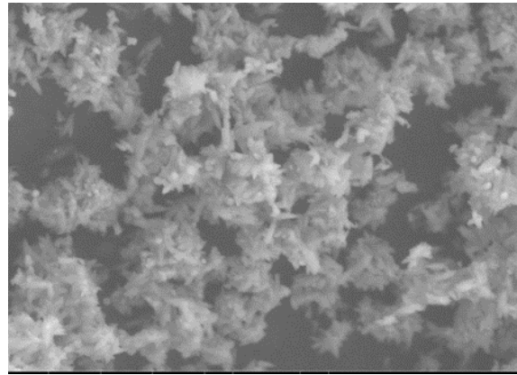
รูปที่ 11 โครงสร้างจุลภาคของนาโนแคลเซียมคาร์บอเนต
