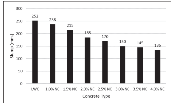
รูปที่ 4 ค่าการยุบตัวของคอนกรีต
