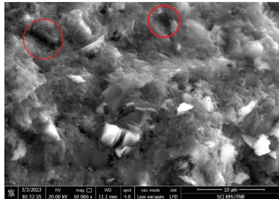
รูปที่ 12 โครงสร้างจุลภาคของคอนกรีตมวลเบา (OPC)
