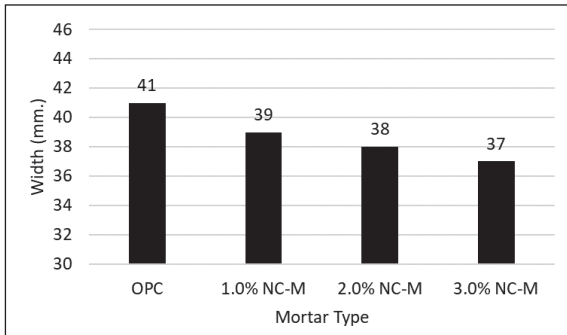
รูปที่ 17 ความกว้างที่เวลาเริ่มต้นในการพิมพ์
