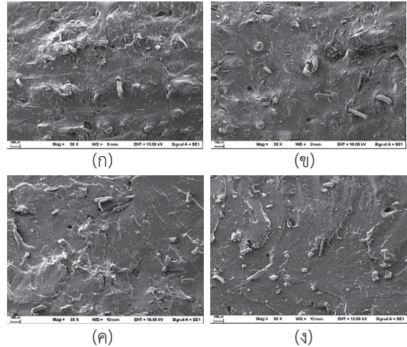
รูปที่ 9 SEM Micrograph ของพื้นผิวการแตกหักจากแรงดึงของยางคอมโพสิต ที่กำลังขยาย 50 เท่า
