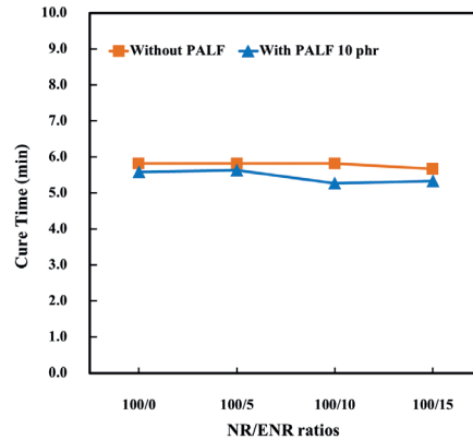
รูปที่ 4 ผลของการเติม ENR25 ที่ ปริมาณต่างๆ ต่อเวลาในการคงรูป (Cure Time)
