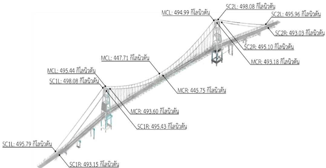
รูปที่ 9 แรงดึงภายในของสายเคเบิลกรณีน้ำหนักบรรทุกคงที่และน้ำหนักบรรทุกจร
