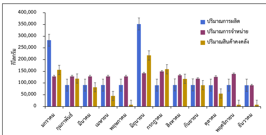
รูปที่ 3 ผลเฉลี่ยของตัวแบบแสดงปริมาณการผลิต ปริมาณการจำหน่าย และปริมาณสินค้าคงคลังที่เหมาะสม
