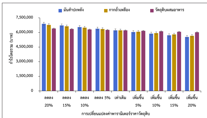
รูปที่ 6 กำไรโดยรวมสูงสุด เมื่อผันแปรค่าพารามิเตอร์ราคามันสำปะหลัง กากถั่วเหลือง และวัตถุดิบผสมอาหาร
