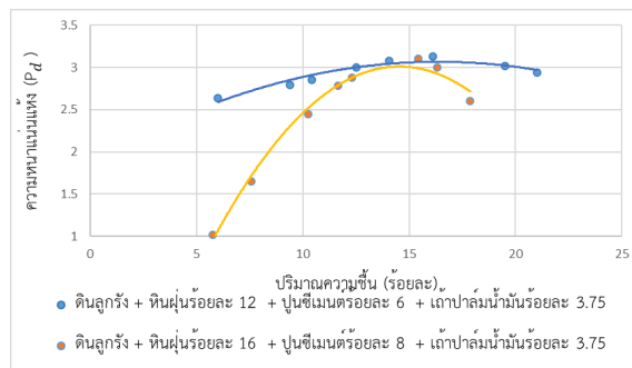
รูปที่ 13 เส้นกราฟการบดอัดแบบสูงกว่ามาตรฐาน (Modified Proctor Test) ของดินลูกรังผสมหินฝุ่น และผสมปูนซีเมนต์ ปริมาณเถ้าปาล์มน้ำมัน 3.75%
