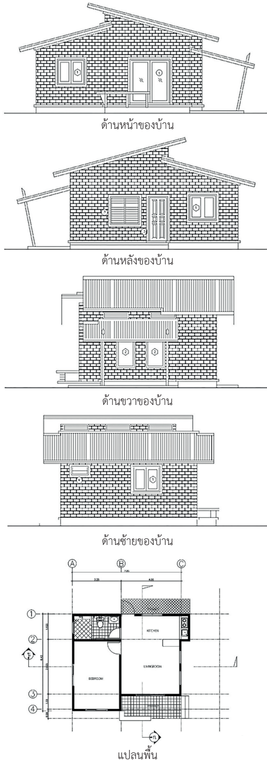
รูปที่ 2 แบบบ้านพักอาศัยต้นแบบที่ใช้ในการวิจัย
