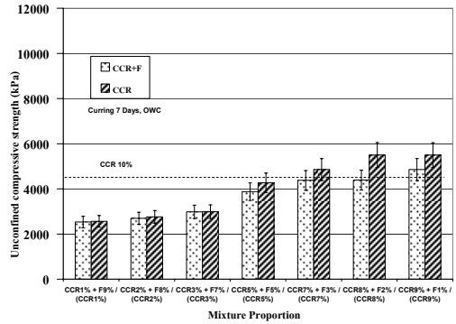
รูปที่ 10 อิทธิพลของเถ้าลอยต่อค่ากำลังอัดแกนเดียวที่กากแคลเซียมคาร์ไบต์อัตราส่วนต่าง ๆ อายุบ่ม 7 วัน
