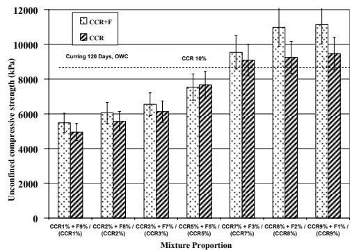
รูปที่ 12 อิทธิพลของเถ้าลอยต่อค่ากำลังอัดแกนเดียวที่กากแคลเซียมคาร์ไบต์อัตราส่วนต่าง ๆ อายุบ่ม 120 วัน
