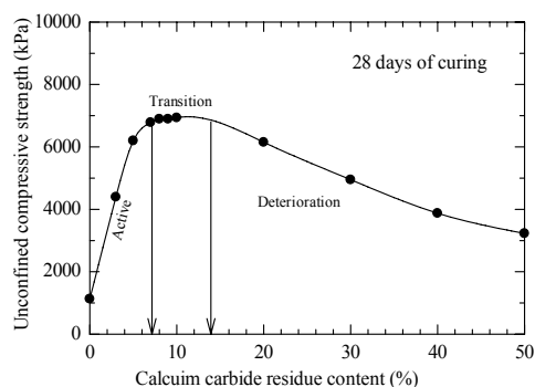
รูปที่ 4 อิทธิพลของกากแคลเซียมคาร์ไบด์ต่อกำลังอัด
