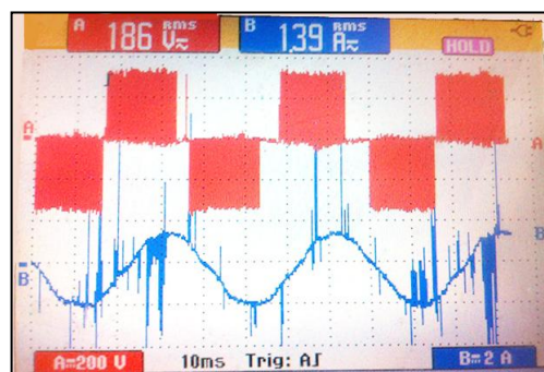
รูปที่ 10 แสดงสัญญาณ PWM และ กระแส ไซนูซอยด์ที่ได้จากการวัด ที่ f_m เท่ากับ 25Hz และ f_s เท่ากับ 12kHz
