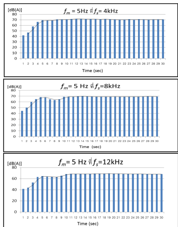
รูปที่ 16 แสดงระดับเสียงที่ f_m = 5 Hz และ f_s ที่ 4, 8, และ 12kHz
