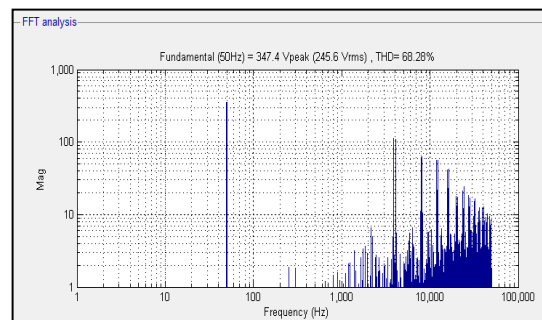
รูปที่ 15 แสดงสัญญาณฮาร์มอนิกที่จำลองการทำงาน ที่ f_m เท่ากับ 25Hz และ f_s เท่ากับ 12kHz
