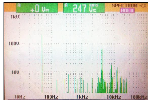
รูปที่ 14 แสดงฮาร์มอนิกที่ได้จากการวัด ที่ f_m เท่ากับ 25Hz และ f_s เท่ากับ 12kHz
