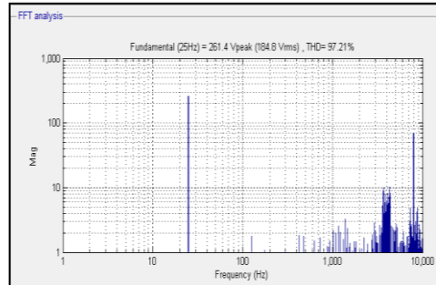
รูปที่ 13 แสดงสัญญาณฮาร์มอนิกที่จำลองการทำงาน ที่ f_m เท่ากับ 25Hz และ f_s เท่ากับ 8kHz
