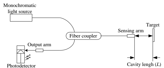
รูปที่ 1 โครงสร้างพื้นฐานของตรวจจับสนใยแก้วนำแสงชนิดฟาบริ-เปโรต์ อินเทอร์เฟอโรมิเตอร์
