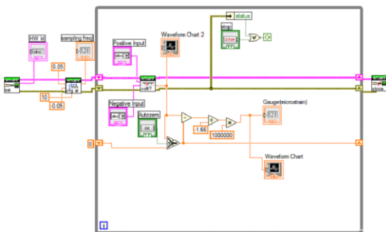
รูปที่ 7 ไดอะแกรมการทำงานของระบบสำหรับวัดค่าความเครียดที่ได้จากगेवदความเครียดมาตรฐาน
