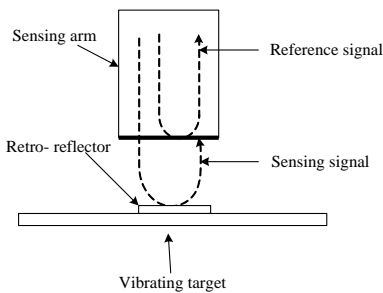
รูปที่ 2 สัญญาณอ้างอิงและสัญญาณวัดที่ถูกกำเนิดภายในตัวตรวจจับฟาบรี-เปโรต์ อินเทอร์เฟอโรมิเตอร์
